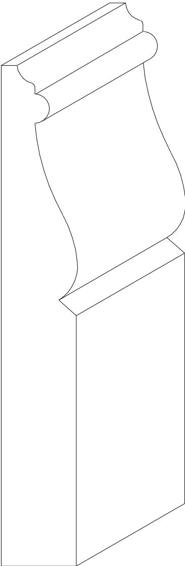
W-585 3/4" x 5"
