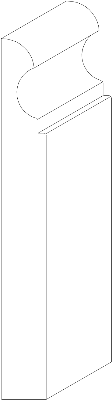
W-571 3/4" x 6"
