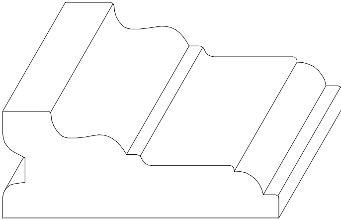
W-1262 1 1/16" x 2 3/4"
