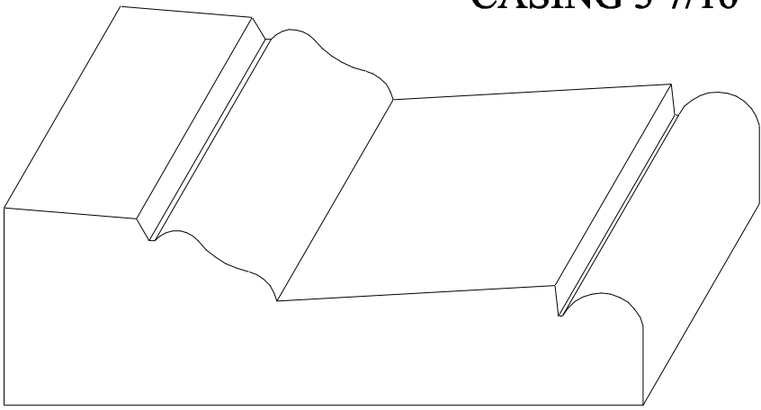
W-1612 1 1/16" x 3 7/16"
