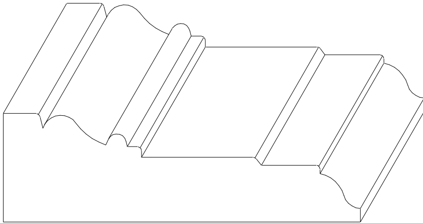
W-890 1 1/16" x 3 1/2"
