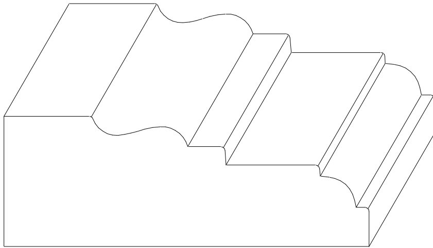
W-1272 1 1/4" x 3 1/2"
