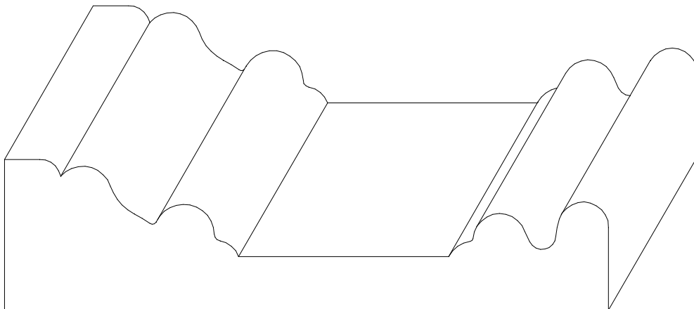
W-573 1 1/16" x 4 1/4"
