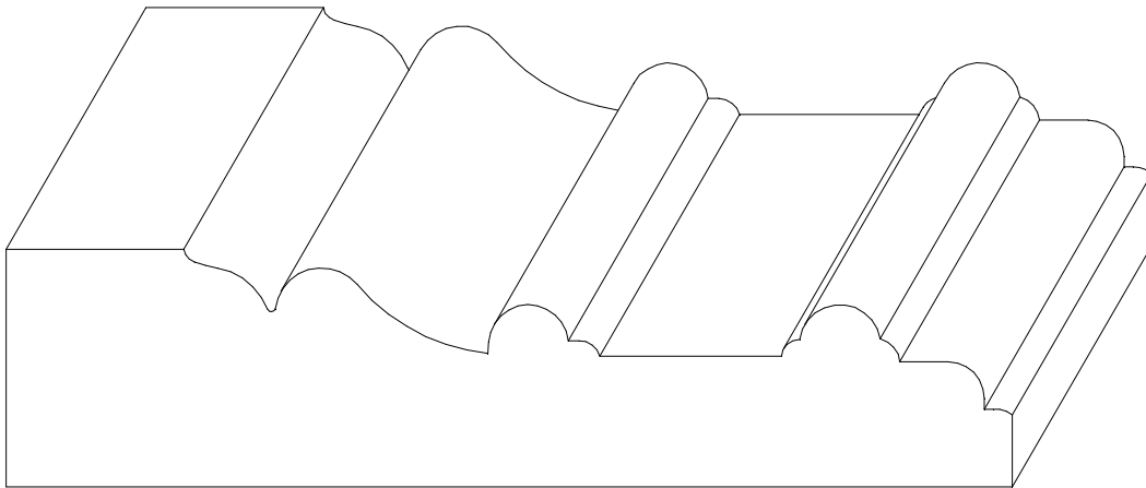
W-1070 1 1/16" x 4 1/2"
