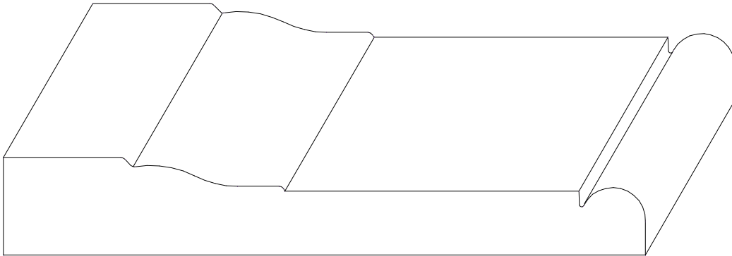
W-318 1 1/16" x 4 1/2"
