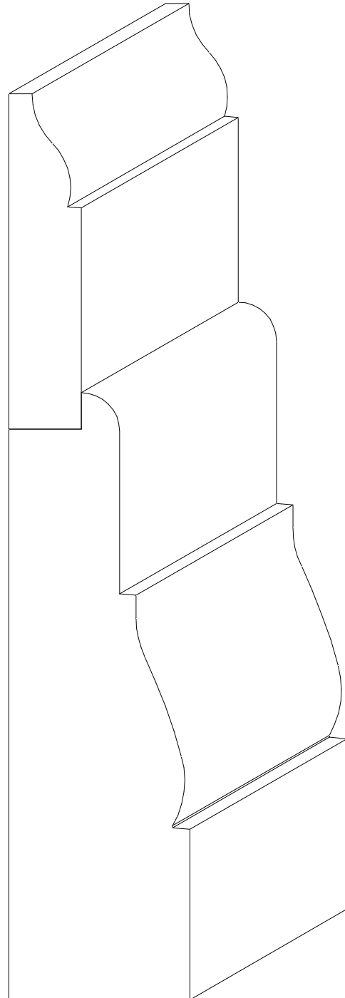
W-870 1 1/4" x 6 1/4"
