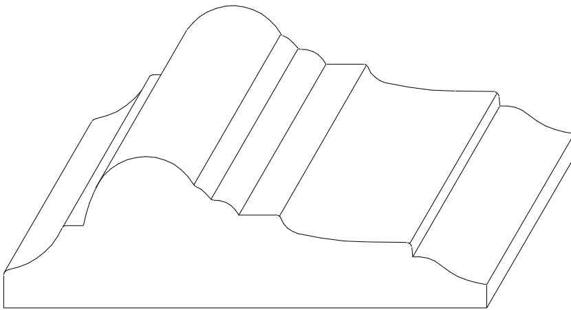
W-1343 1 1/16" x 3 7/16"
