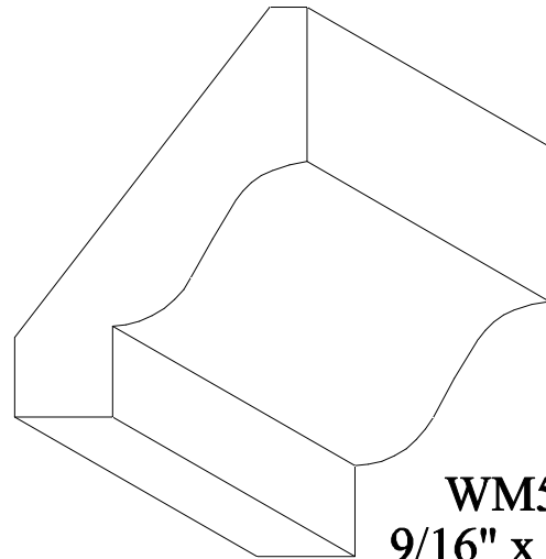
WM58 9/16" x 2 3/4"
