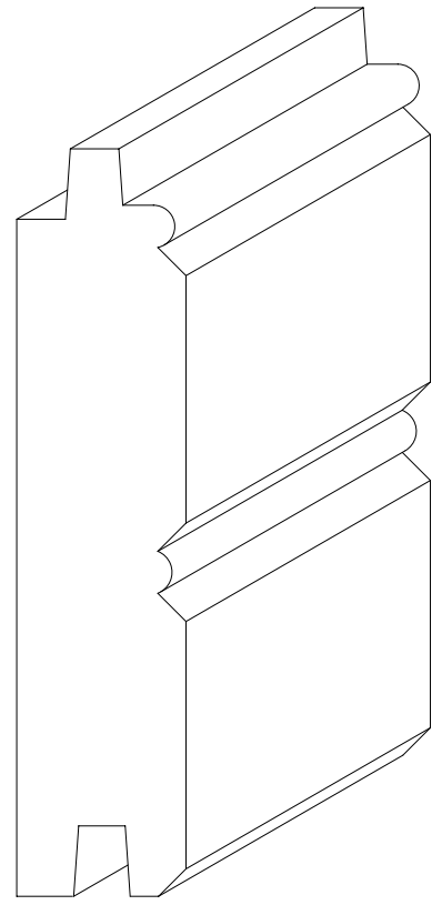
W-357 3/4" x 3 1/16" FACE
